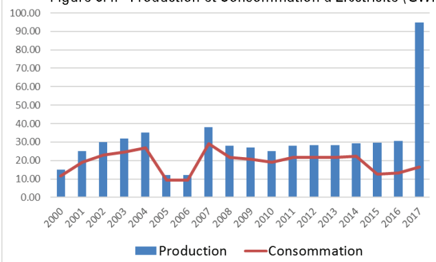
Figure 3.4. - Production et Consommation d'Électricité (GWh)
