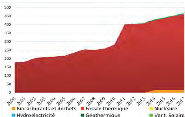
Figure 3.3. - Production d'Électricité par Source (GWh)
