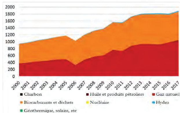
Figure 3.1. - Approvisionnement total en énergie primaire (ktpe)
