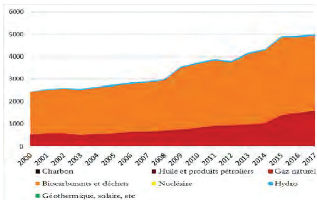
Figure 3.1. - Approvisionnement total en énergie primaire (ktpe)
