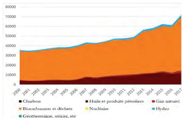
Figure 2.3. - Production d'Électricité par Source (GWh)
