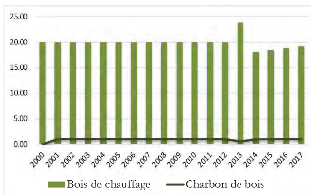
Figure 3.6. - Production de Bois de Chauffage et de Charbon de Bois (1000 tonnes)
