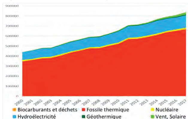
Figure 2.3. - Production d'Électricité par Source (GWh)
