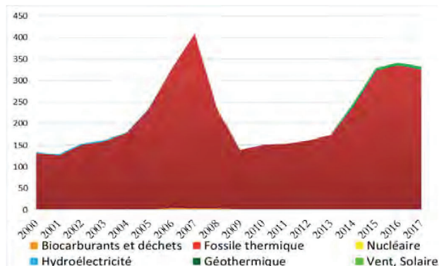
Figure 3.3. - Production d'Électricité par Source (GWh)
