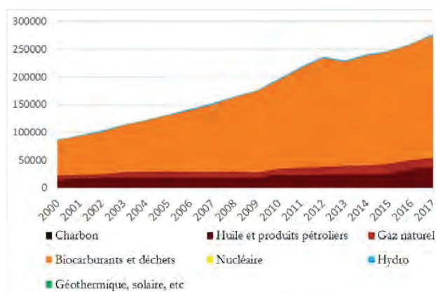
Figure 2.3. - Production d'Électricité par Source (GWh)
