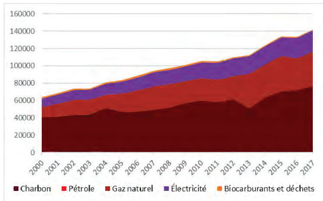
Figure 2.2. - Consommation Finale Totale (ktpe)
