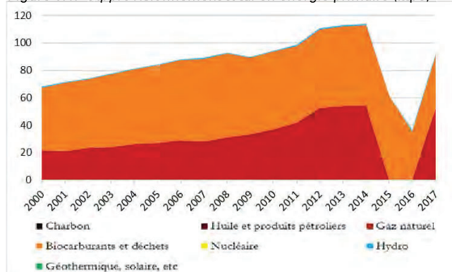
Figure 3.1. - Approvisionnement total en énergie primaire (ktpe)
